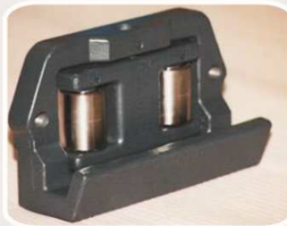
Presilhas inferiores com Roletes de Rolamento de Agulha.
